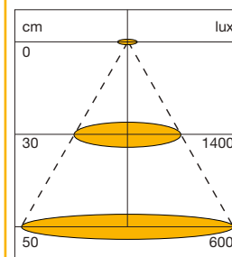
Dijagram raspodjele svjetlosti
