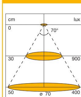
Dijagram raspodjele svjetlosti
