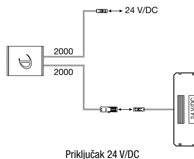
Priključak 24 V/DC
