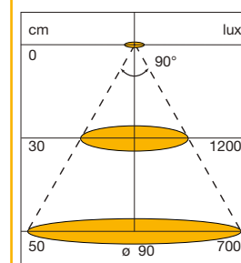
Dijagram raspodjele svjetlosti
