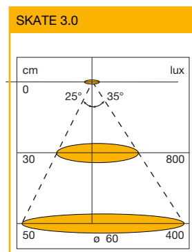
Dijagram raspodjele svjetlosti
