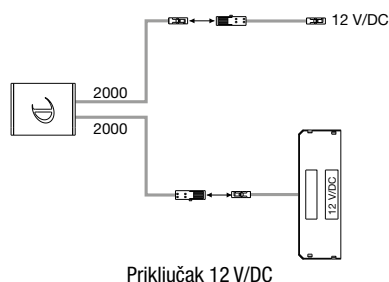
Priključak 12 V/DC
