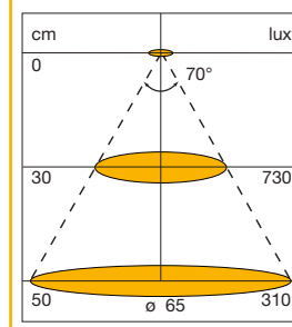
Dijagram raspodjele svjetlosti
