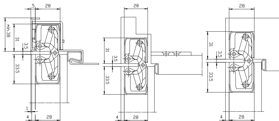
Montaža na čeličnom okviru
