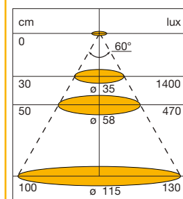
Dijagram raspodjele svjetla
