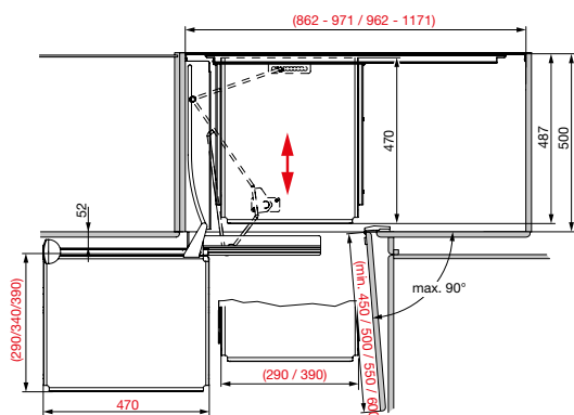
Slika pokazuje smjer izvlačenja na desno
