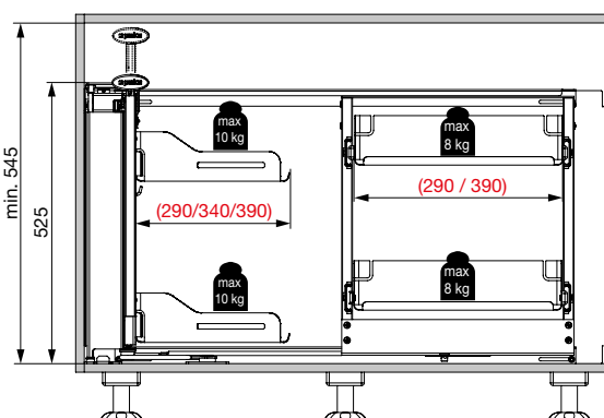
Slika pokazuje smjer izvlačenja na desno
