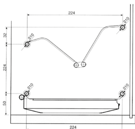
Slika bušenja Ø 10 i 10 mm dubina
