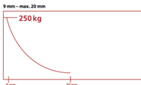
Sila stezanja / udaljenost od ruba
