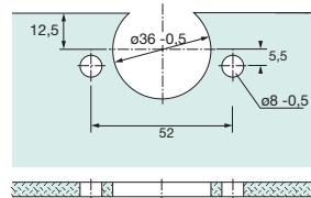
Šablona stak.vrata za čašicu T 22
