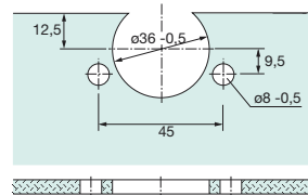
Šablona stak.vrata za čašicu TB 22
