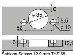
Šablona Sensys 12,9 mm THS 55
