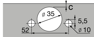
Šablona bušenja Sensys tanka vrata VV 52
