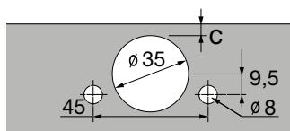
Šablona bušenja Sensys 12,9 mm TB 55
