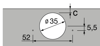
Šablona bušenja Sensys 165° 8657 TH 52
