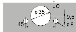
Šablona bušenja Sensys 165° 8657 TB52
