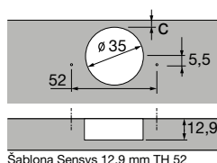
Šablona Sensys 12,9 mm TH 52
