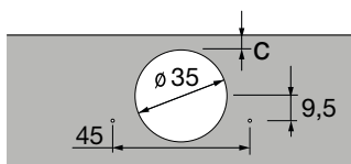
Šablona bušenja Sensys tanka vrata ŠV52
