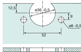
Šablona stak.vrata za čašicu T22/9
