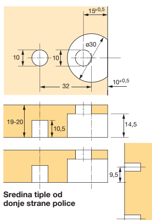
Slika bušenja Polica 19-20 mm
