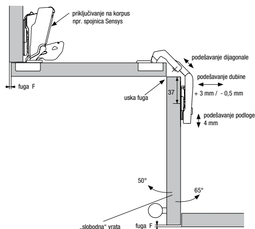
Šablona Sensys 12,9 mm TH 52
