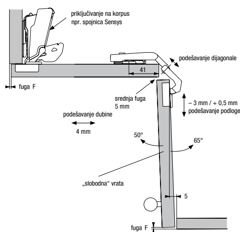
Šablona Sensys 12,9 mm THS 55
