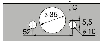
Šablona bušenja Sensys 165° 8657 TH 52
