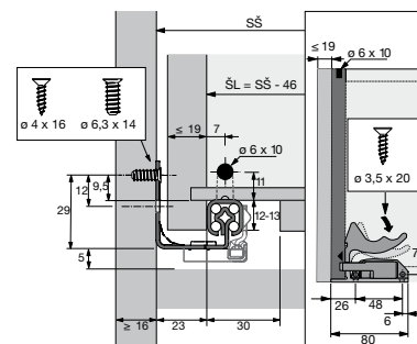
Dno s utorom
