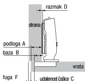
Šablona bušenja Sensys tanka vrata ŠV52
