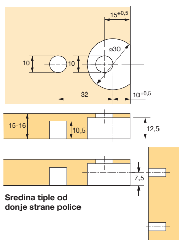
Slika bušenja Polica 15-16 mm
