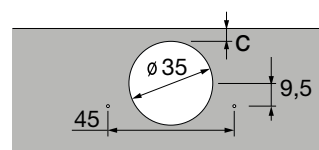
Šablona bušenja Sensys 165° 8657 TB52
