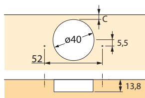
Mjere bušenja T 22/40
