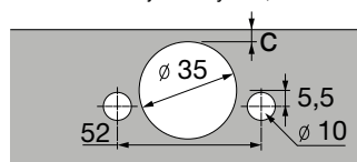
Šablona bušenja Sensys 12,9 mm TH 52
