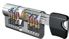
Ugradbeni cilindri keyTec RPE
